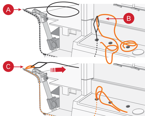
Einfädelposition
