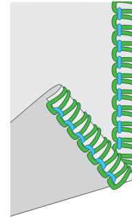
2-Faden-Rollsaum
